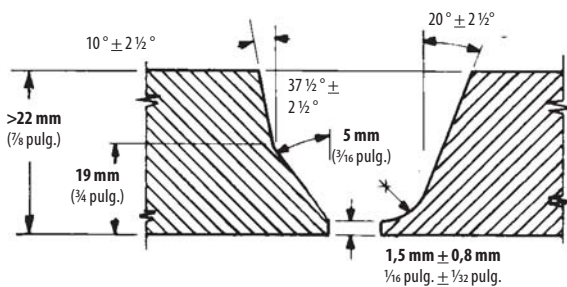
(b) Espesor de la pared más de 22 mm ( \frac{7}{8} \text{ pulg.} )
