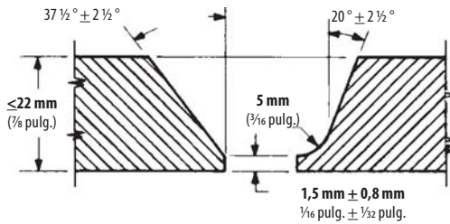
(a) Espesor de la pared de 6 mm a 22 mm, inclusive ( \frac{1}{16} \text{ pulg.} - \frac{7}{8} \text{ pulg.} )
