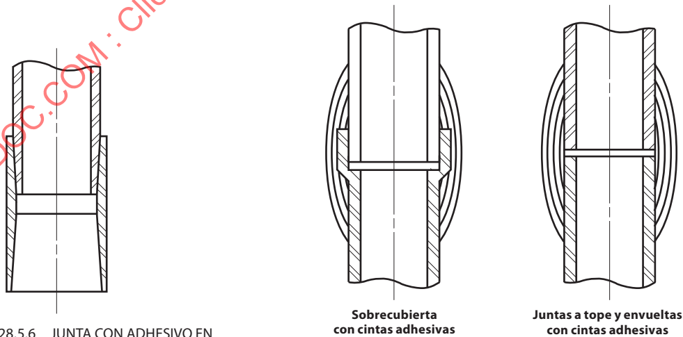
FIGURA A328.5.7 JUNTAS ENVUeltas CON CINTAS ADHESIVAS EN TUBERÍA TERMOESTABLE
