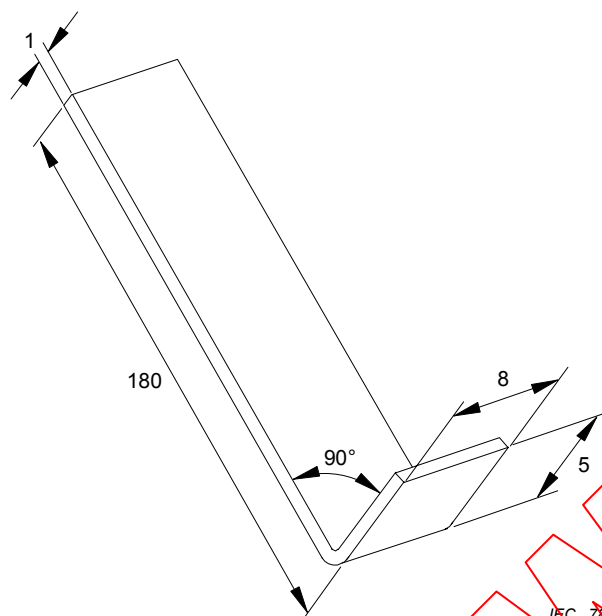
Figure 4 – Crochet d'épreuve
