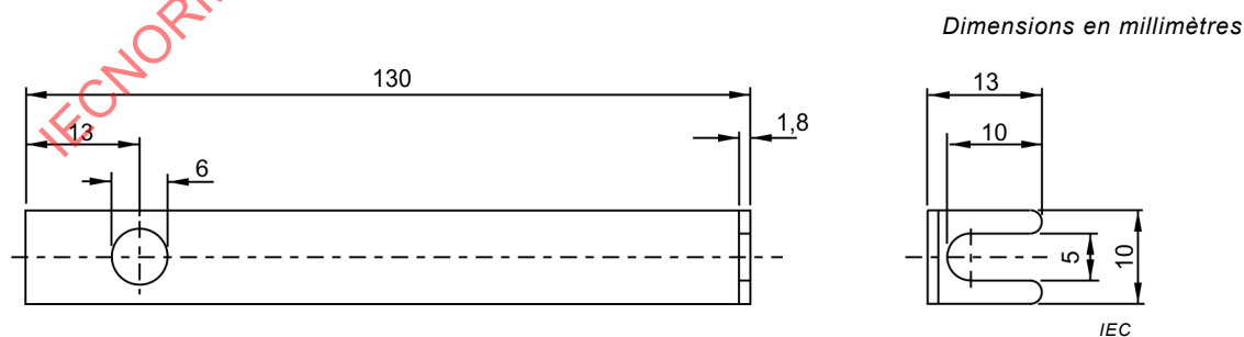
Figure 4 – Languette d'essai
