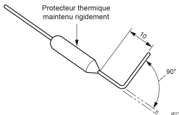
Étape 1: Pliage
