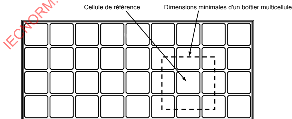
Figure 2 – Cellule de référence unique dans un boîtier multicellule
