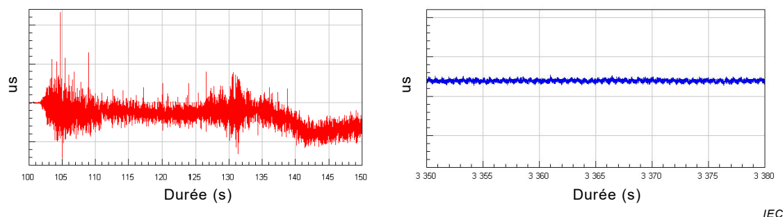
Figure 6 – Signal de jauge de contrainte au démarrage et à pleine charge sur une aube de turbine Francis
