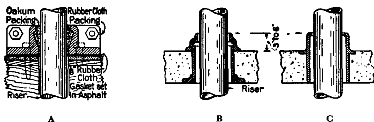
Fig. 3068. Watertight Riser Sleeves.
